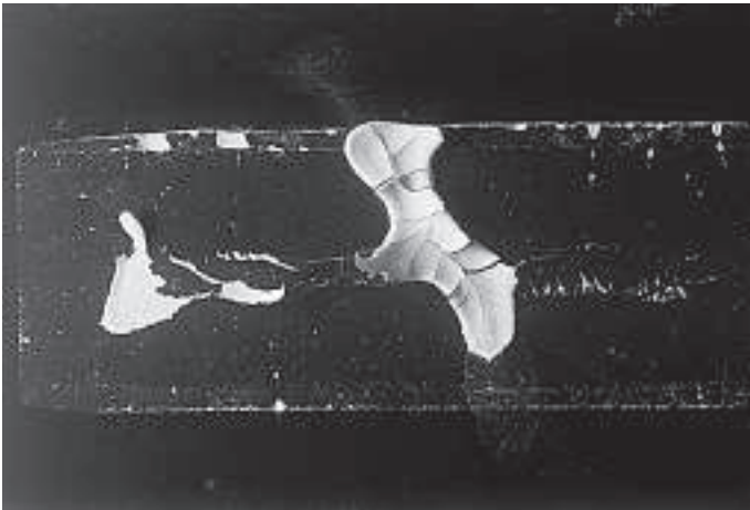
5 Reines Kieselsol haftet nicht auf einem PVC-Untergrund (links). Stabilisiertes Kieselsol, verwendet in einer Sol-Silikatfarbe, führt hingegen zu guten Verarbeitungseigenschaften (rechts). (Foto: Keimfarben)
