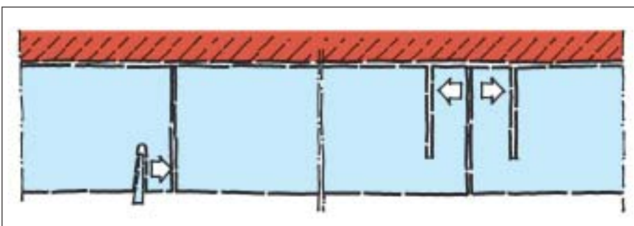
3 Gegen offene Stossfugen in Wärmedämmplatten helfen Keile (links) oder Schlitze auf der Rückseite (rechts).
