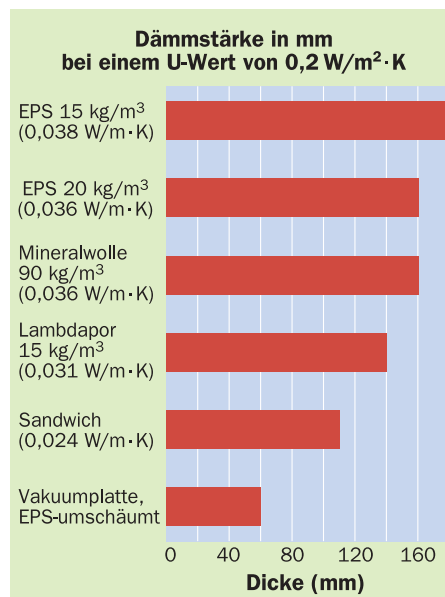
7 Die Dicke verschiedener Wärmedämmplatten auf einem Modulbackstein von 175 mm Stärke bei konstantem U-Wert von 0,2 W/m 2 K. Wenn die Dämmstärke wieder abnimmt, können konstruktive Anschlussdetails kostengünstiger gelöst werden.
