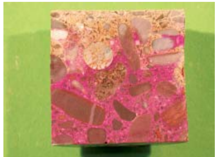
Mit einem Indikator lässt sich die Karbonatisierungstiefe einer Betonprobe bestimmen.
